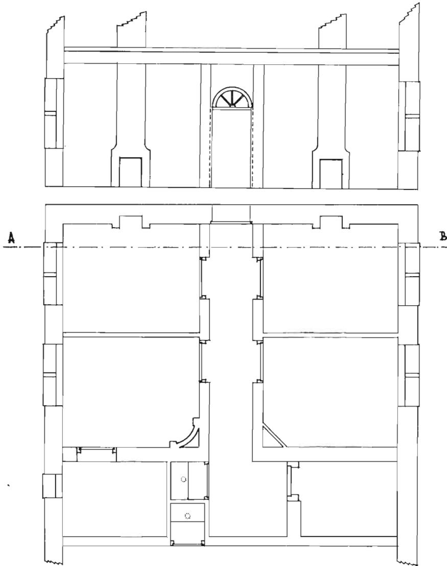
Afb. 9. Indeling van het raadhuis, begane grond. Naar een „plattegrond- teekening der interigten kazerne voor de Brigade Marechaussé”, 1847. (tekening Dienst Gemeentewerken)
