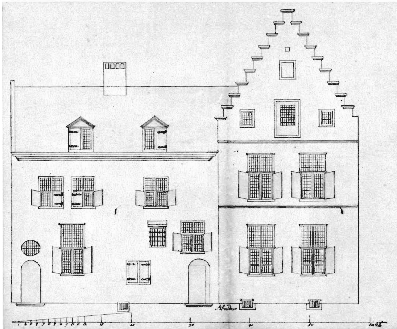
4. Gevel van het huis Nazareth (anno 1762), waarin de schuilkerk van de Nieuwstraat was gevestigd.
