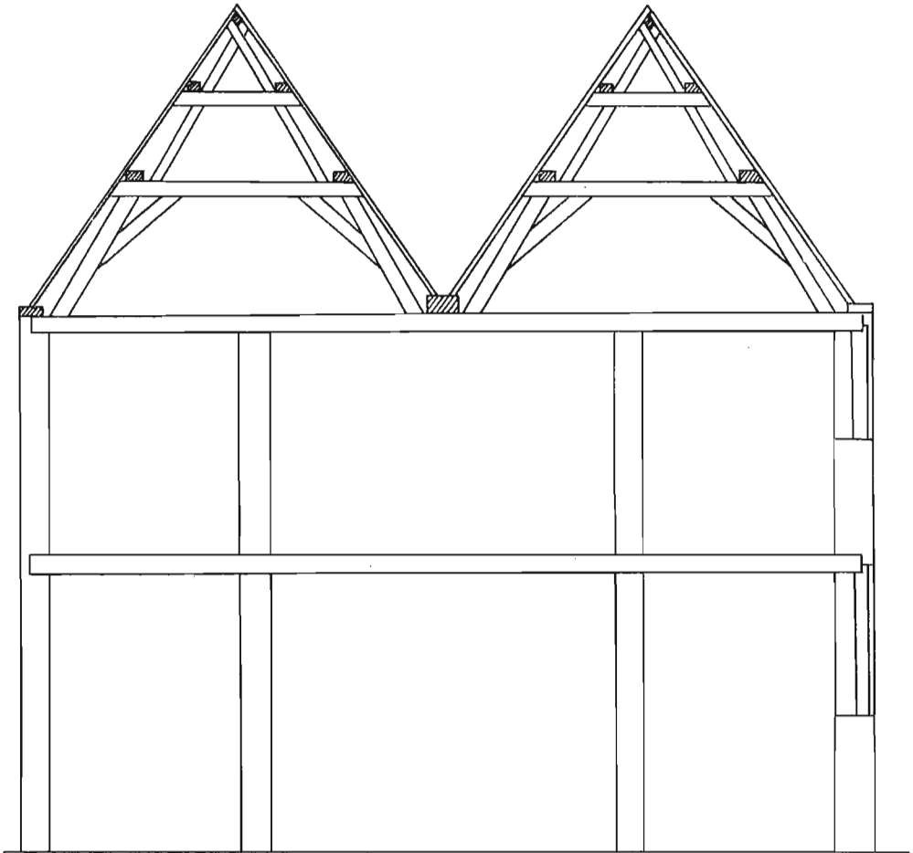
Doorsnede van de in 1716 voltooide kerk aan de Waterstraat. De constructie is duidelijk berekend op de aanleg van galerijen.
