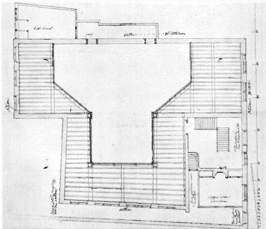
6-7. Plattegonden der galerijen in de schuilkerk aan de Nieuwstraat vóór en na de verbouwing van 1762. De samenstelling van de kerkruiimte uit twee pakhuizen laat zich hieruit gemakkelijk aflezen.
