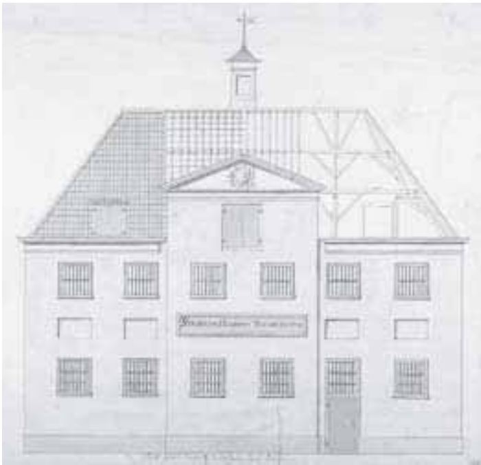
1. Het tuchthuis, gevel aan de Oude Vest. Ontwerptekening door A. Canters, 1775.
