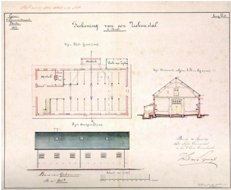
20. 'Teekening van een Ziekenstal te Breda', Genie 1877. (NL-HaNA 4.OPG inv. nr. B403)
