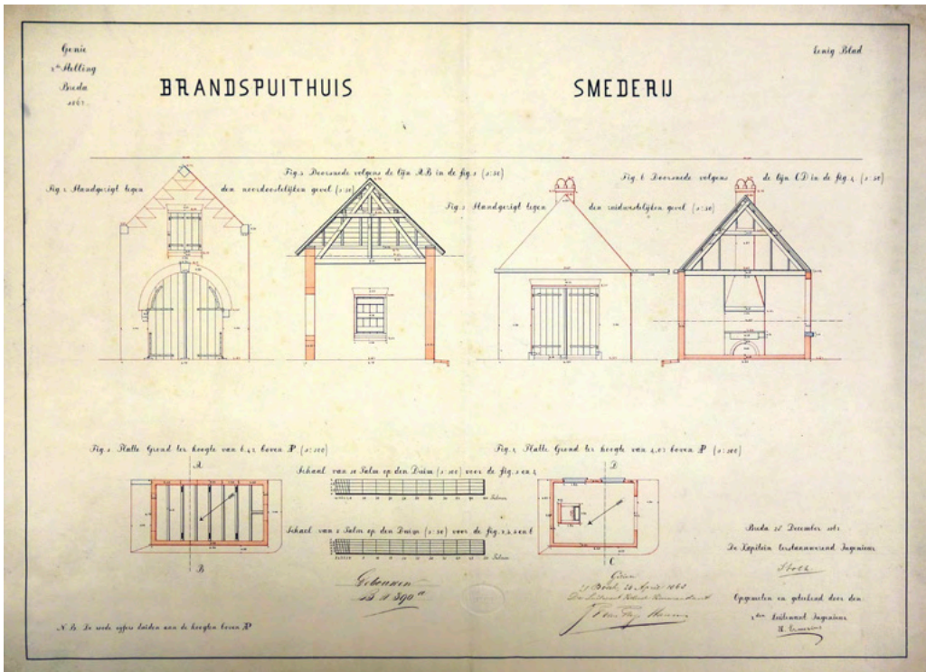
13. Opmeting van brandspuithuis en smederij, Genie 2e stelling Breda 1867. (NL-HaNA 4.OPG inv. nr. B390)
