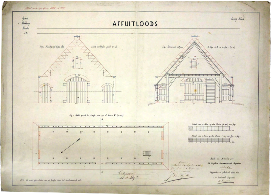
12. Opmeting van de Affuitloods door de Genie 2 e stelling, Breda 1867. (NL-HaNA 4.OPG inv. nr. B389)
