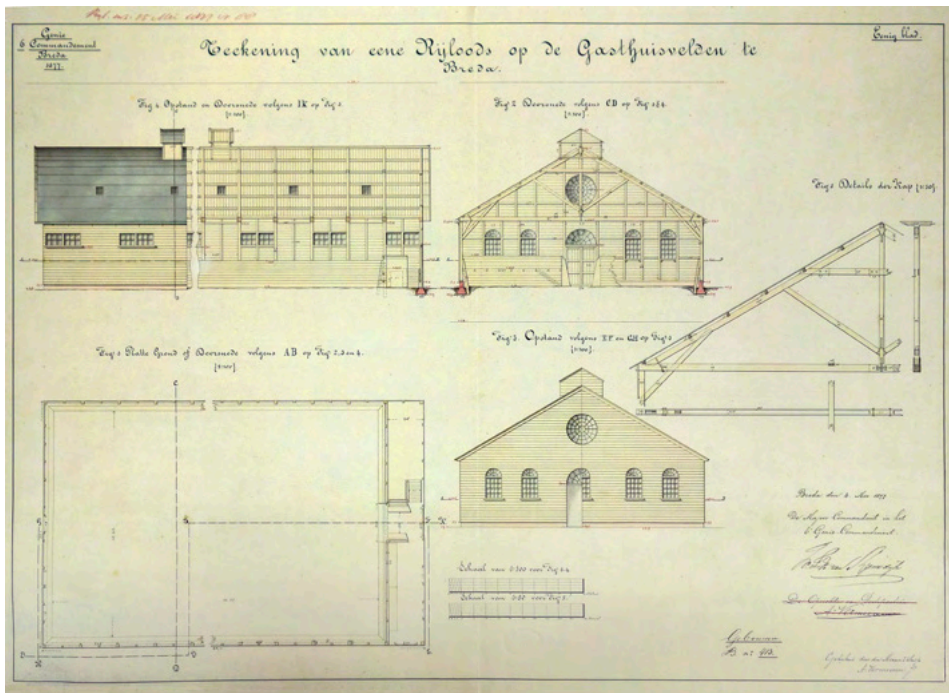
19. 'Teekening van ene Rijloods op de Gasthuisvelden te Breda', Genie 1877; (NL-HaNA 4.OPG inv. nr. B413)
